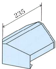
剣先
